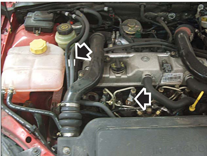
Label en kop verstuiver zie pijl in afbeelding - vooraanzicht
