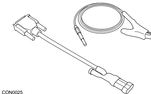
A2C59512069 - kabel Fiat/Alfa/Lancia OBD
