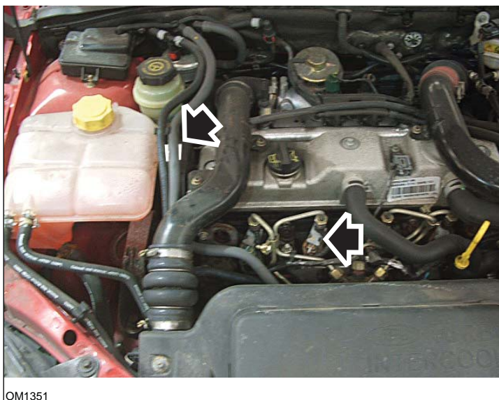
Zdjęcie pokazuje naklejkę z kodami wtryskiwaczy i głowicę wtryskiwacza – widok z przodu.
