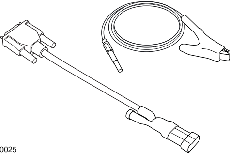
A2C59512069 - Cablu OBD Fiat/Alfa/Lancia
