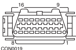
Conector de diagnoză J1962
