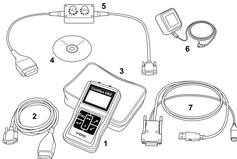
Комплект ContiSys OBD
